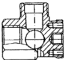
15 Крестовина переходная
