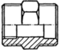
17 Ниппель переходной
