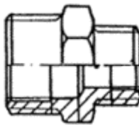
18 Муфта
