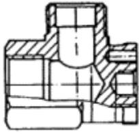
9 Тройник Н
