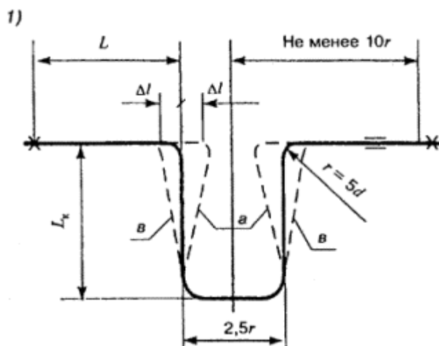
Рисунок 10 - Диаграмма для определения удлинения труб
