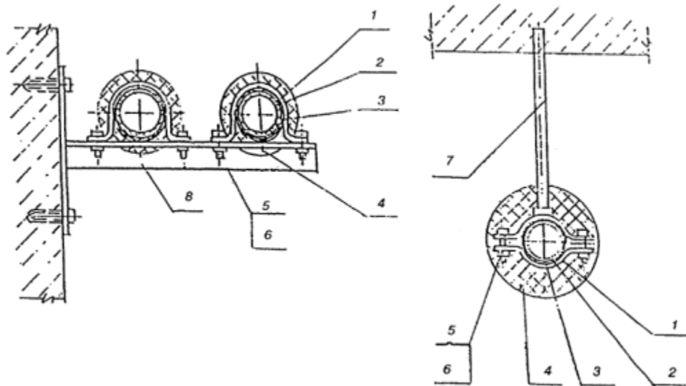
Рисунок 17 - Крепление труб к стенам и перегородкам
