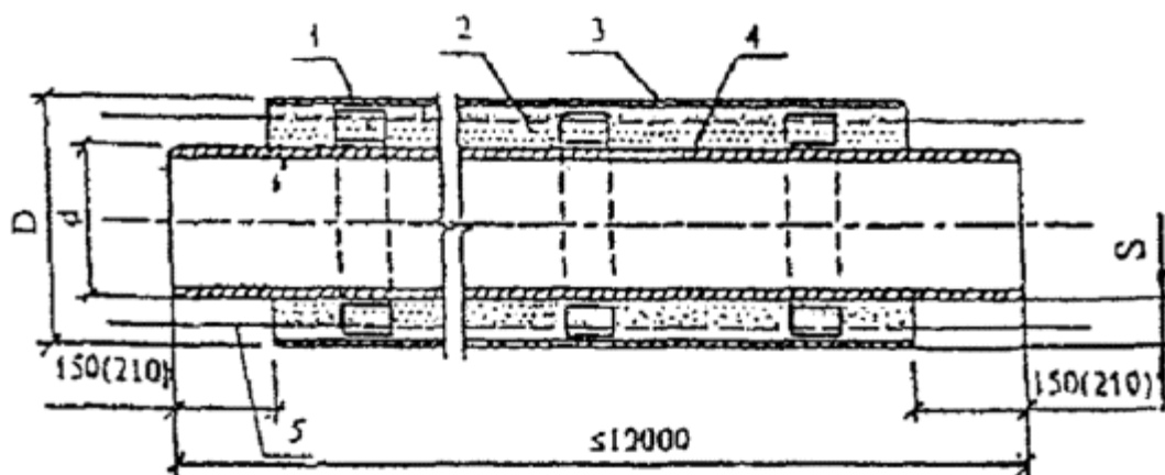
Рис. 1. Индустриальная конструкция труб с ППУ-ПЭ изоляцией
